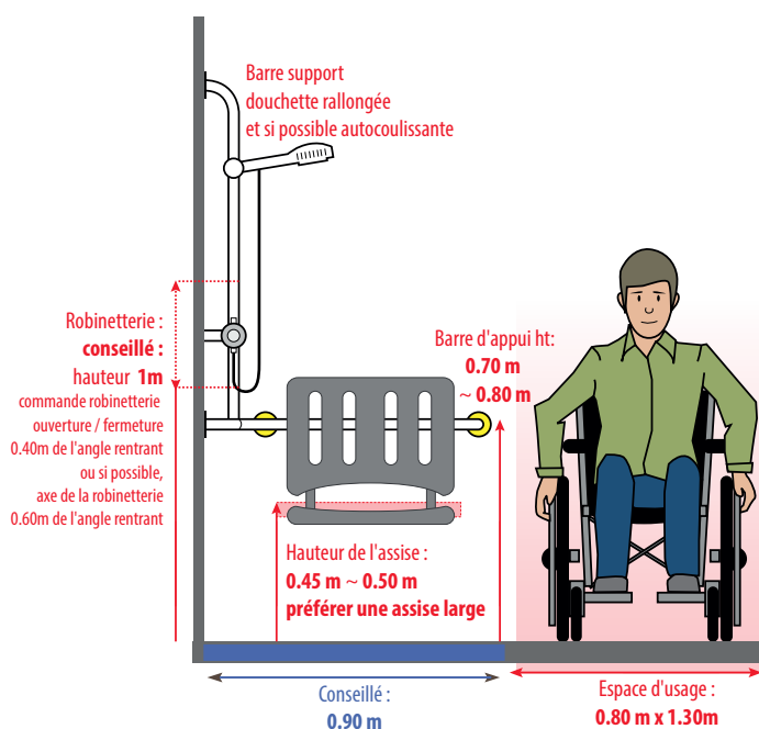
Exemple d'adaptation d'une salle de bain avec douche de plain pied
