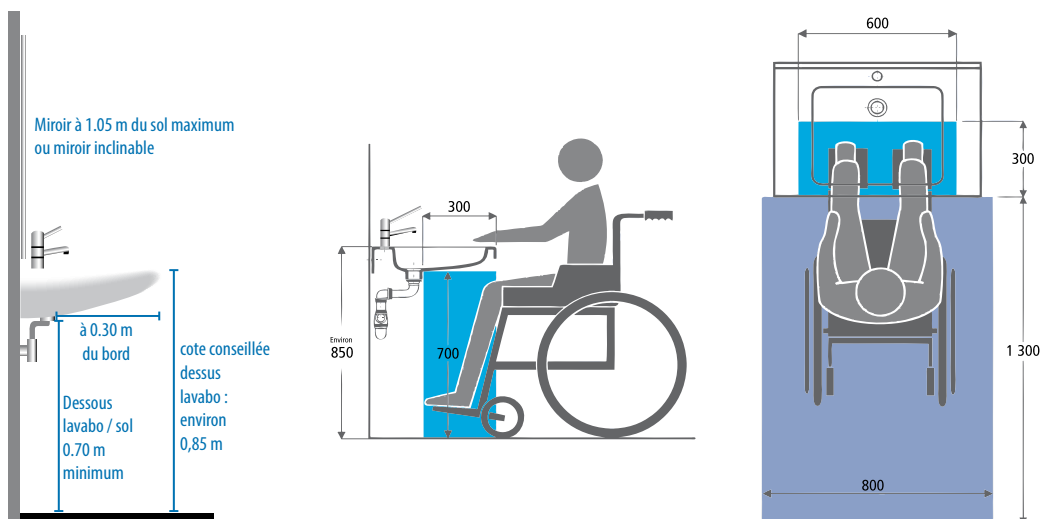
Adaptation d'un lavabo pour une personne en fauteuil roulant
