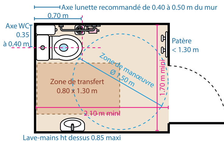
Exemple d'agencement technique d'un bloc WC
